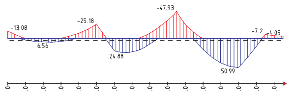
Grenzmomente wahlweise mit/ohne Umlagerung
