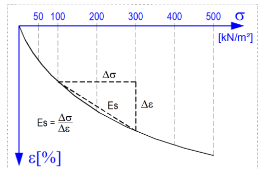
Bild 2: Nichtlineares Baugrundverhalten
